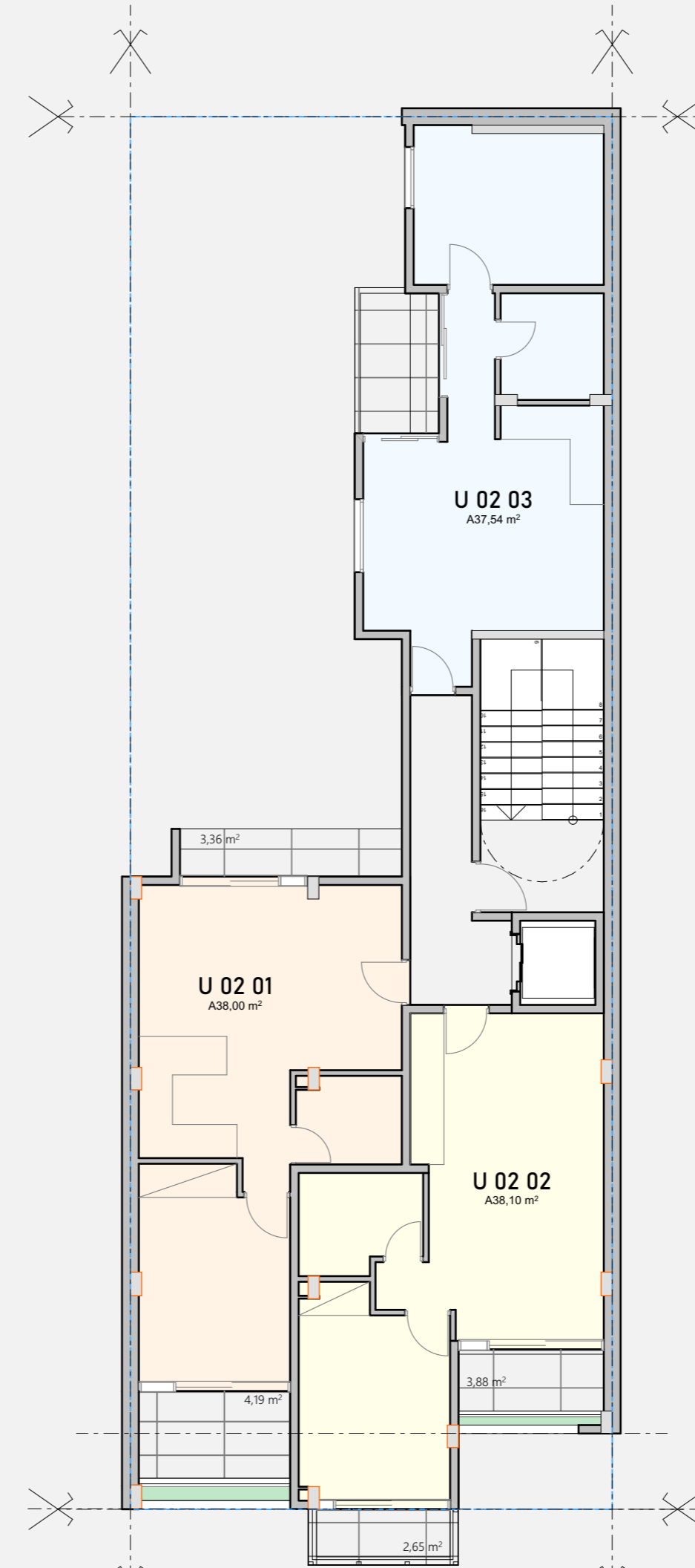
PISO 2 1:100
