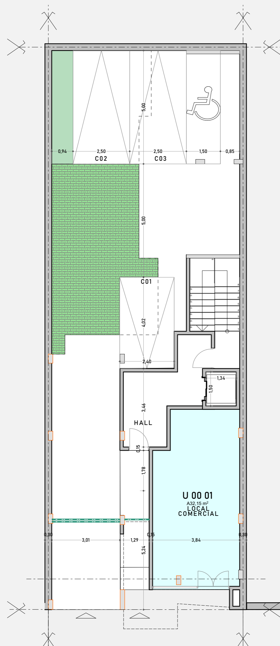
PLANTA BAJA 1:100
